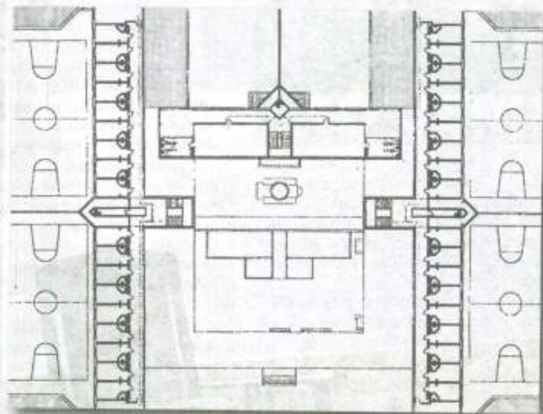
Κάτοψη των νέων φυλακών υψίστης ασφαλείας Ναυπλίου
